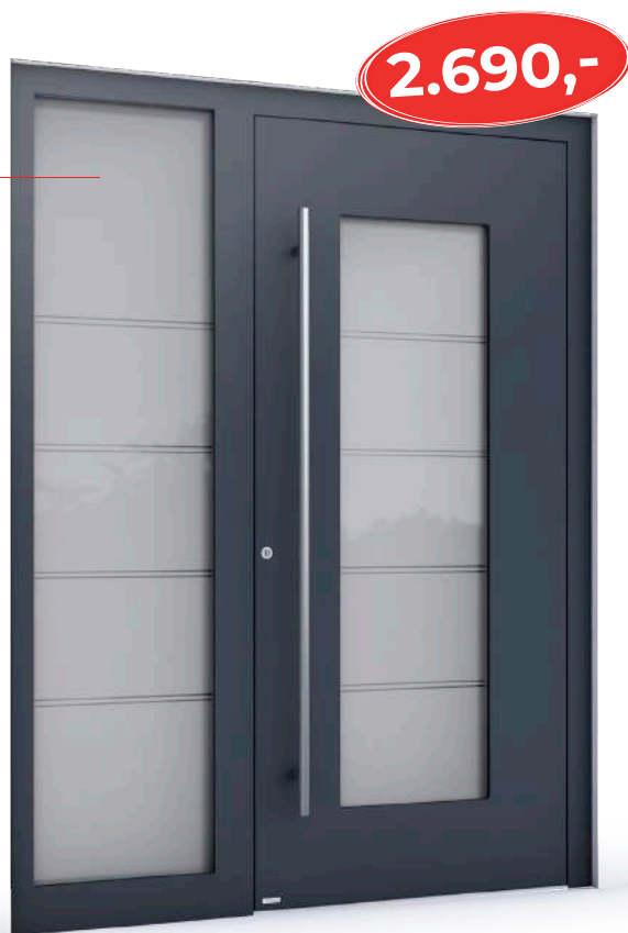
PCA 1
